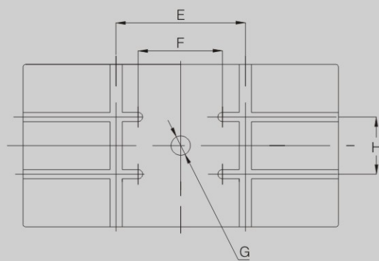
上工作台 Upper worktable
