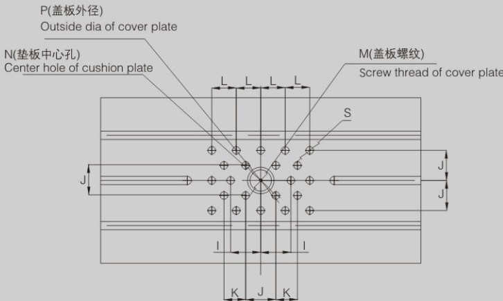
下工作台(II款) Bottom worktable II
