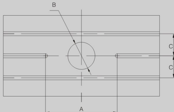
下工作台(I款) Bottom worktable I
